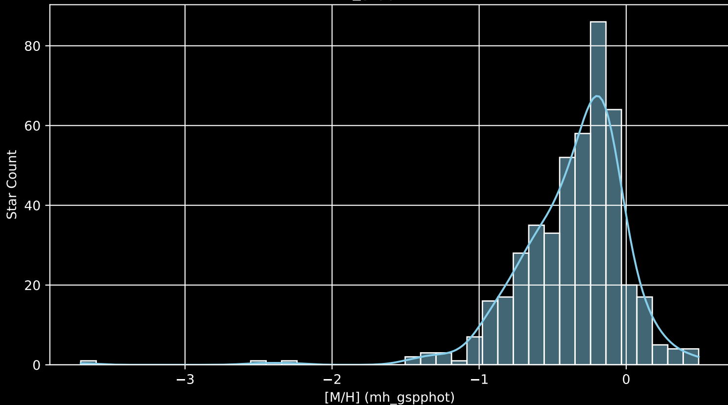
GALAH DR4 Field: [6781] [M/H] (mh_gspphot) (n= 458)
