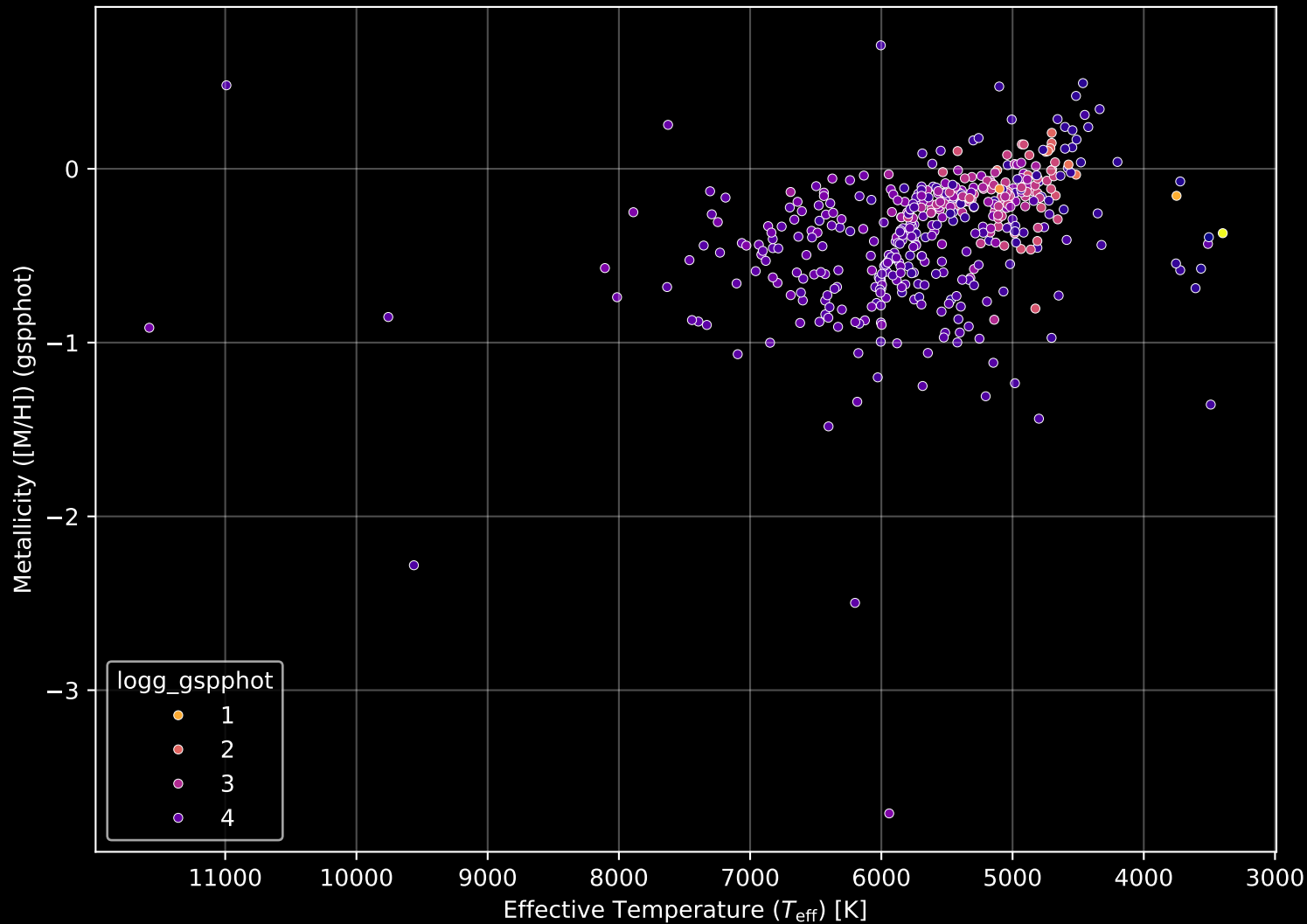
GALAH DR4 Field: [6781] Stellar Population Parameters (n= 459)
