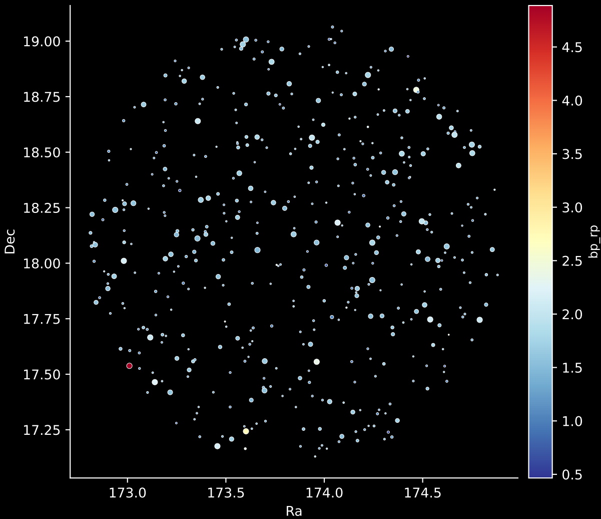
GALAH DR4 Field: [6781] Stars: 459
