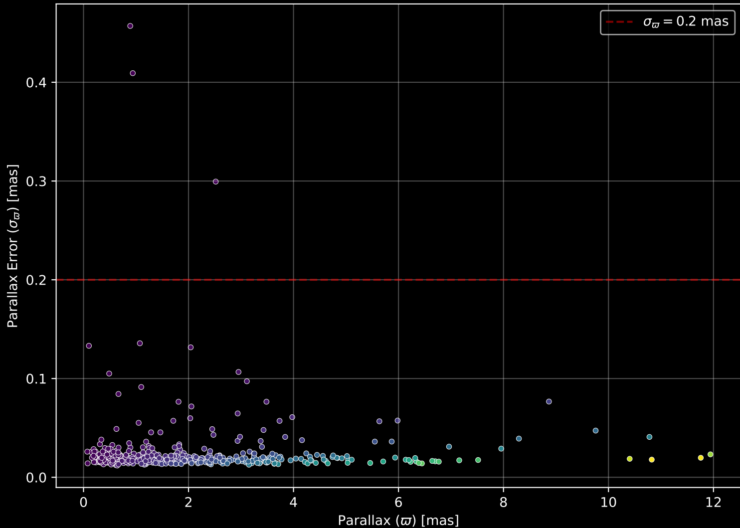
GALAH DR4 Field: [6781] Parallax Quality (n= 459)
